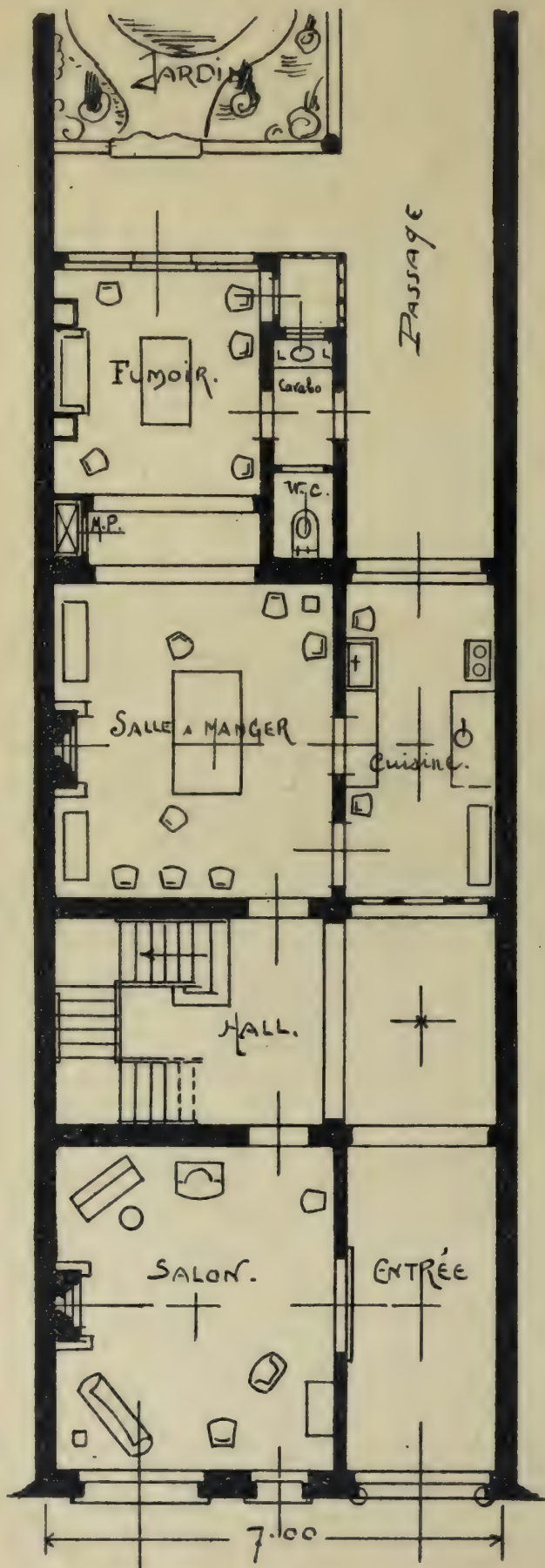
REZ-DE-CHAUSSÉE.
